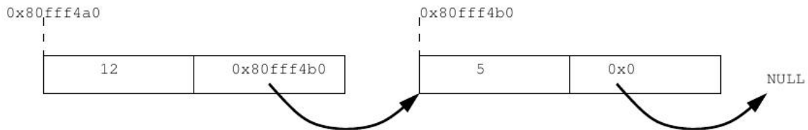
FIGURE 6 – Une liste chaînée
