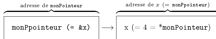
FIGURE 3 – Assignment de monPointeur par l'adresse de x (dans les boîtes, on représente la valeur stockée par la case mémoire ; au-dessus, l'adresse de la case mémoire ; la flèche nous aide juste à visualiser le lien).
