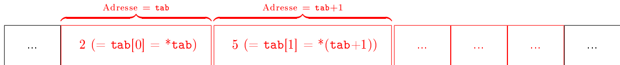
FIGURE 4 – Représentation mémoire de tab
